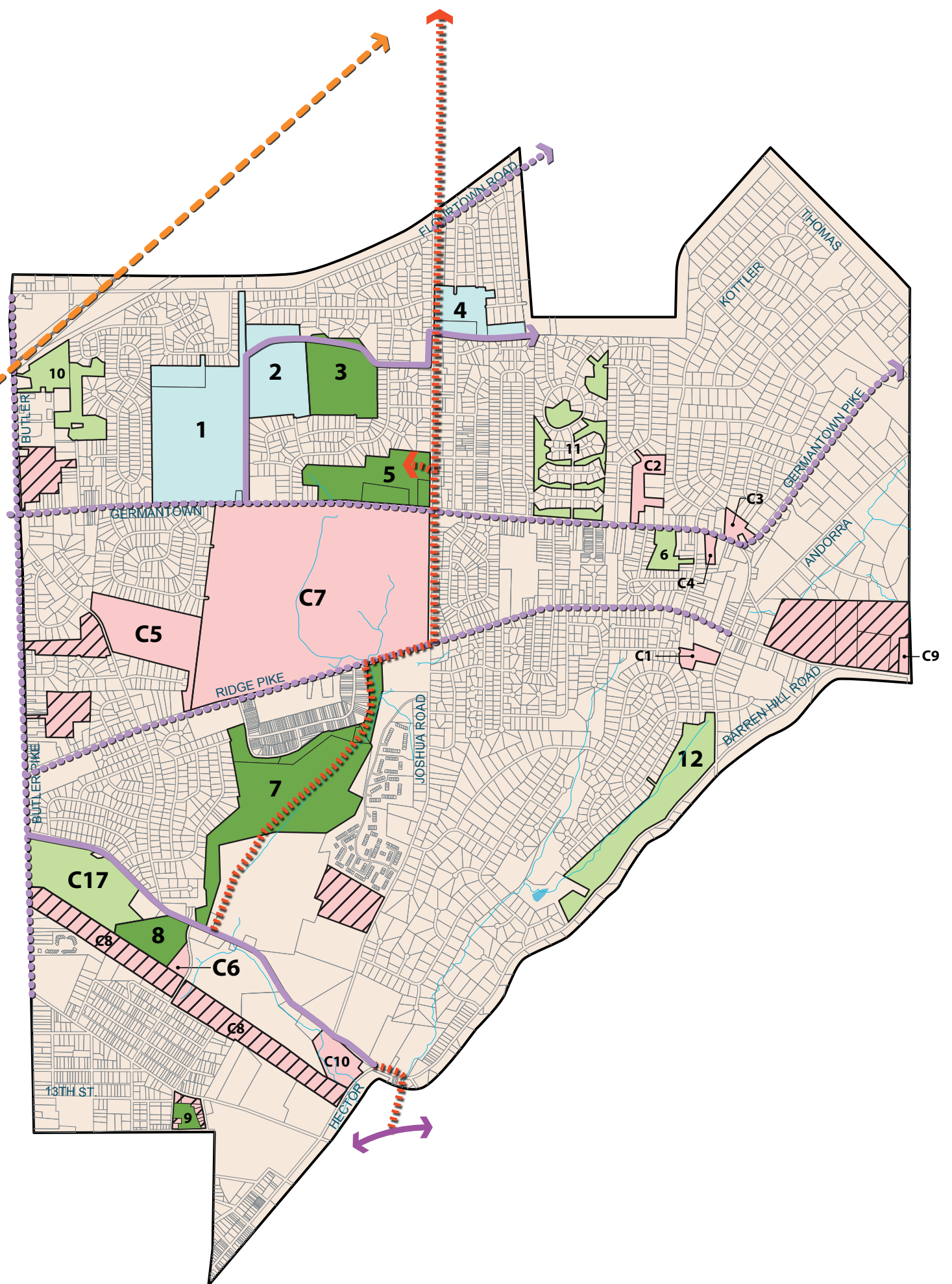
Context Map
